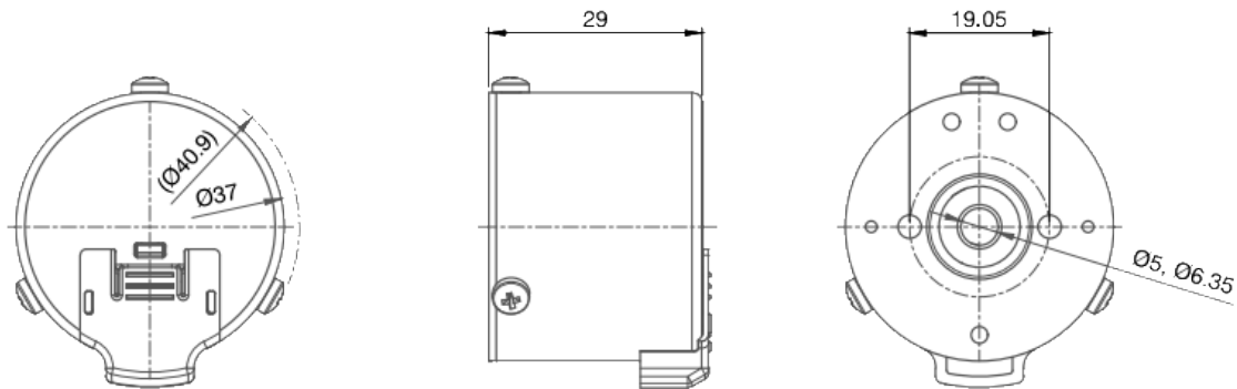
Abb. 1: Maße in mm.
