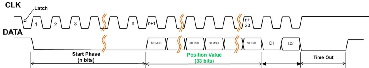
Abb. 2: Datentransfer per SSI.
